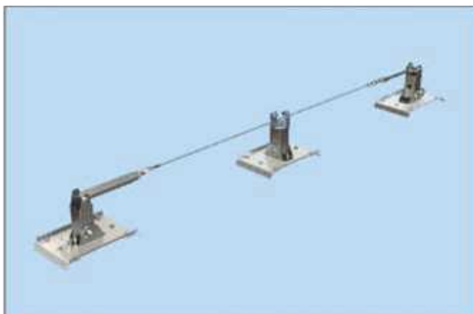
Linea vita permanenti realizzate con cavi, dissipatore, tenditore e ancoraggi in acciaio
