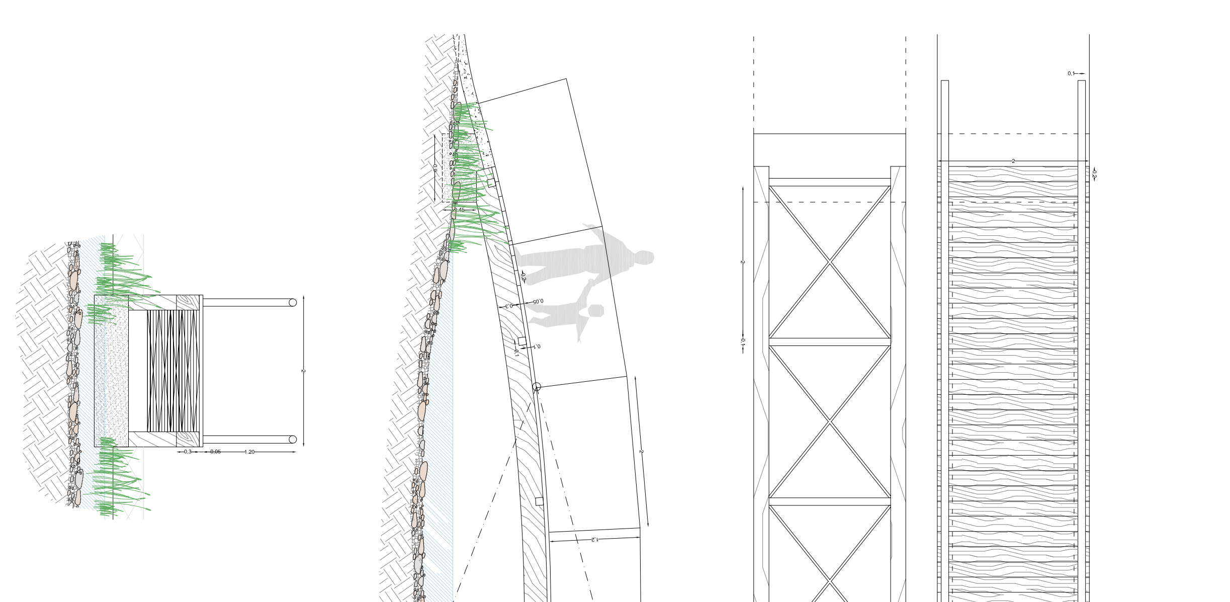
PROSPETTO, SEZIONI rapp. 1:50
