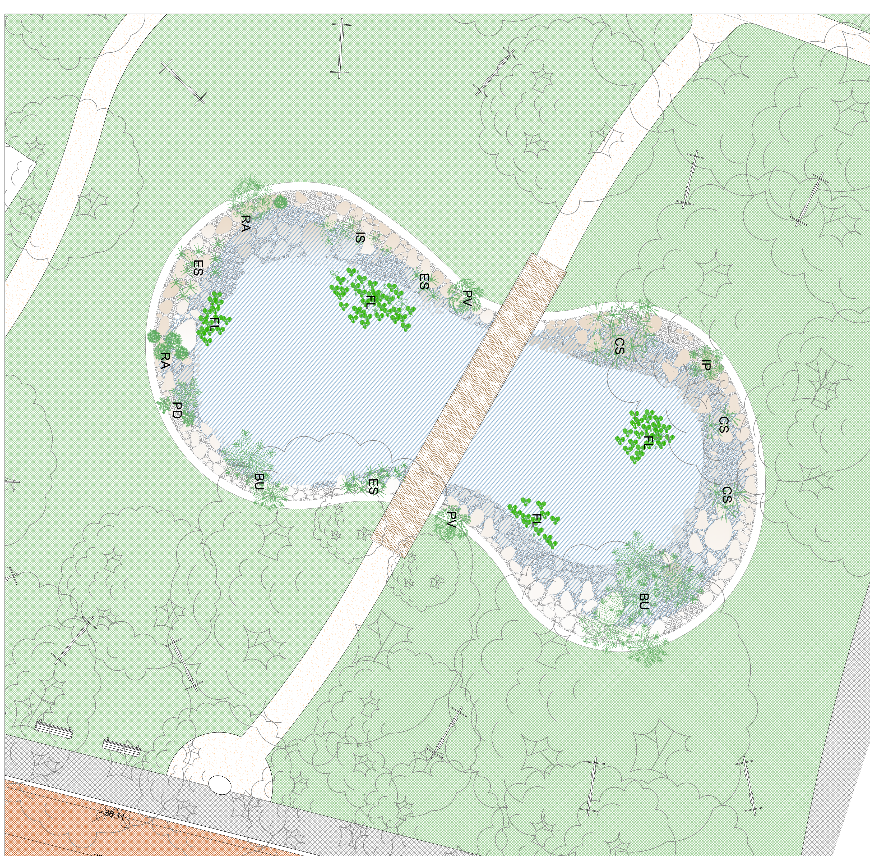
PIANTA rapp. 1:100
