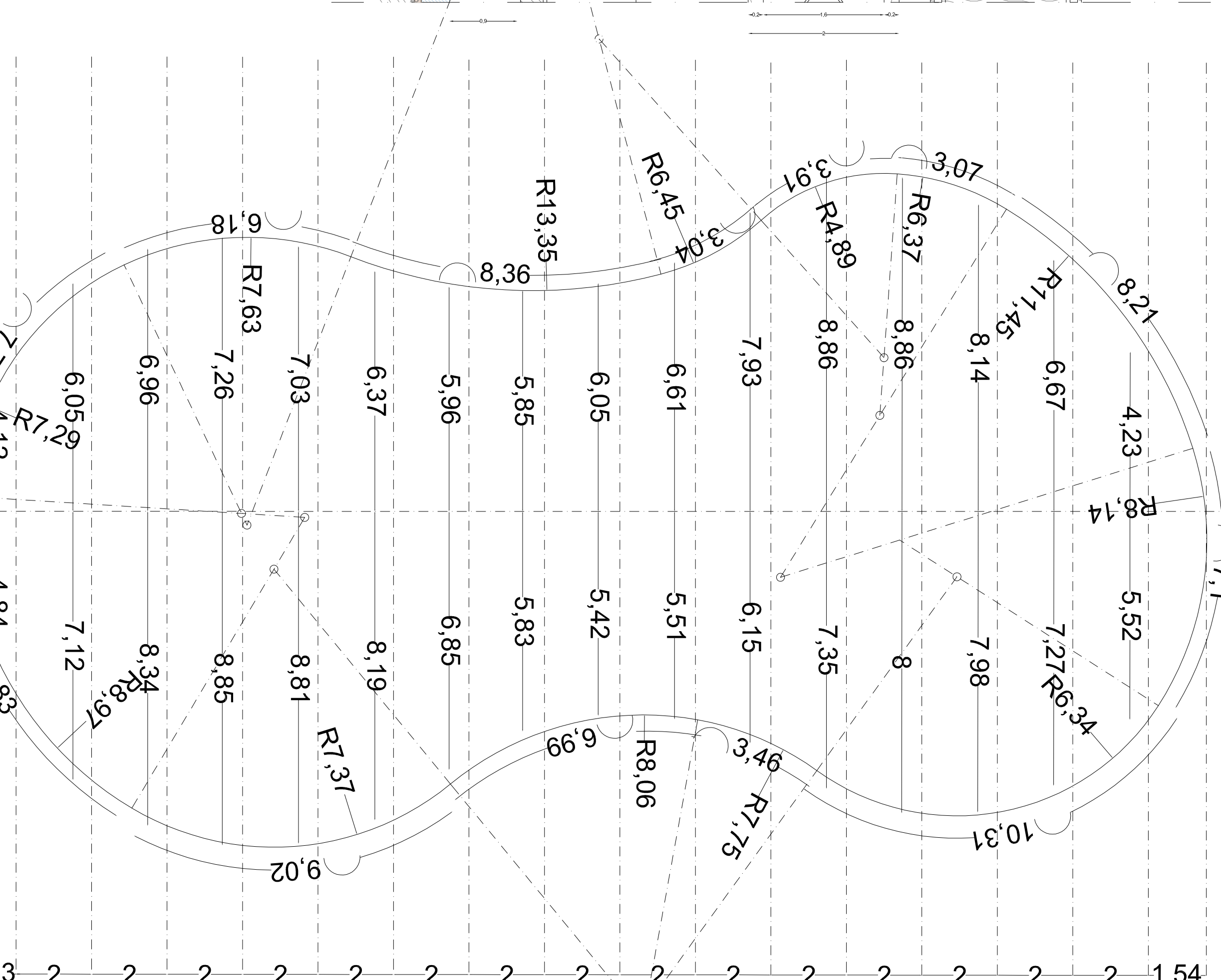
COSTRUZIONE GEOMETRICA rapp. 1:100
