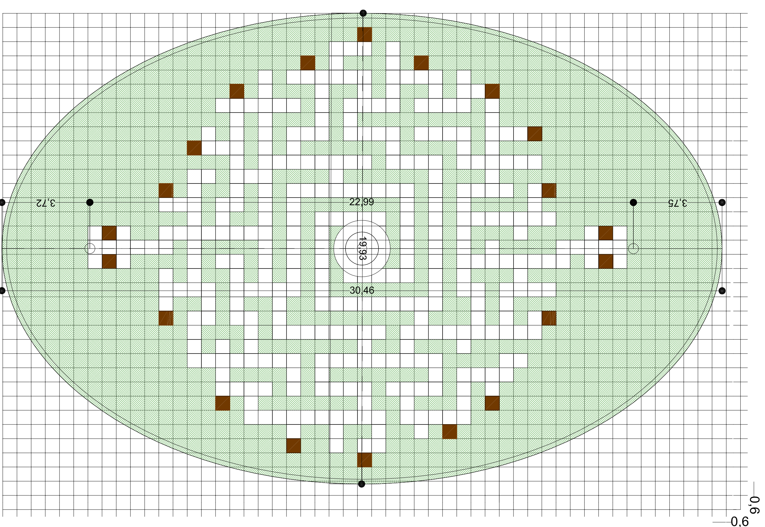
COSTRUZIONE GEOMETRICA rapp. 1:100
