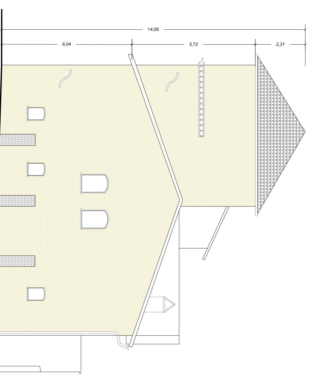
PROSPETTO EST
