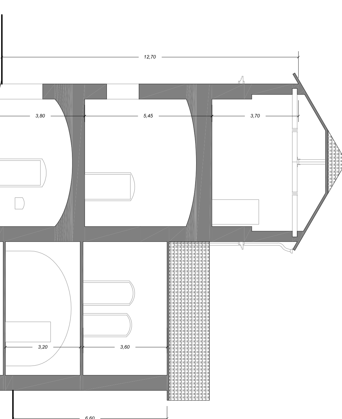
SEZIONE AA
