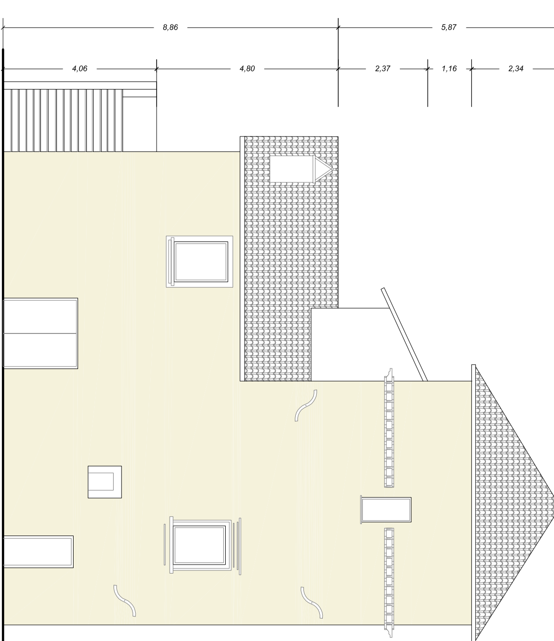
PROSPETTO SUD
