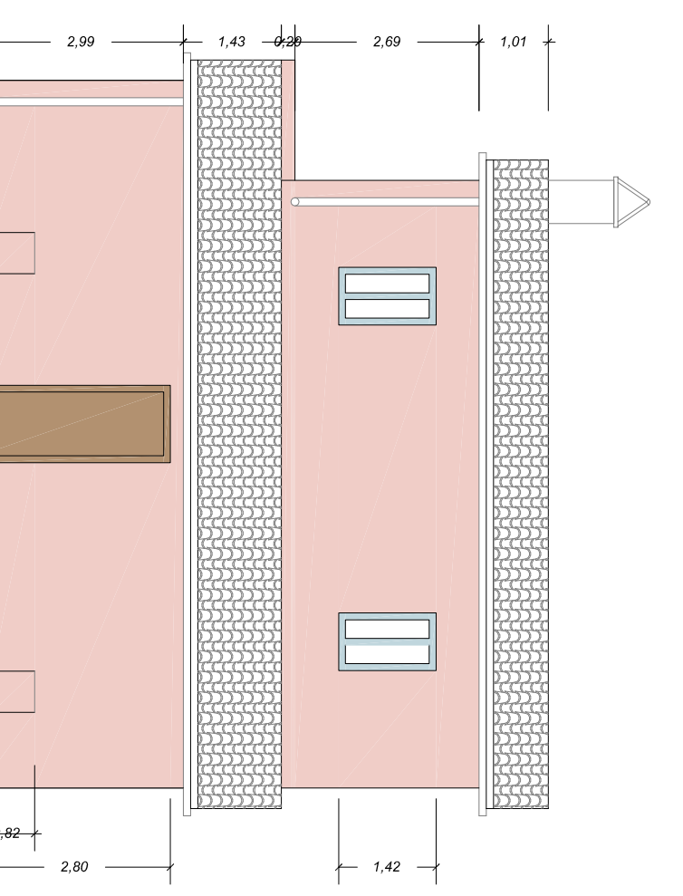
PROSPETTO NORD
