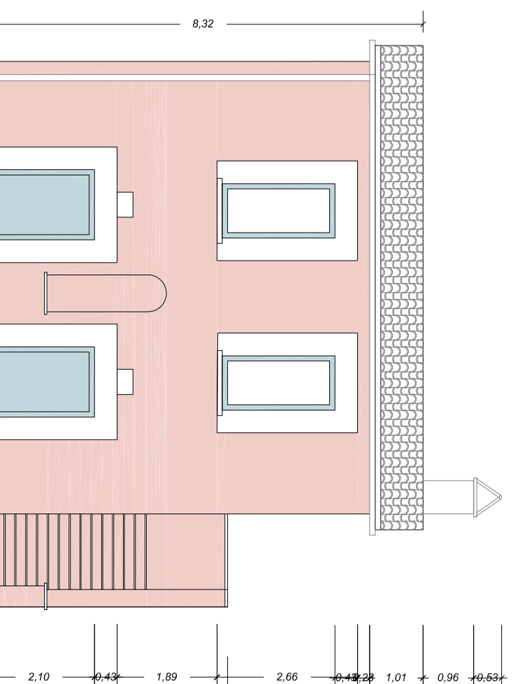
PROSPETTO SUD
