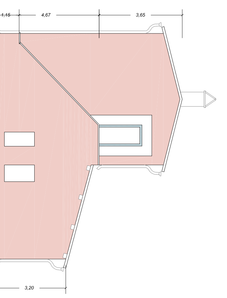
PROSPETTO EST
