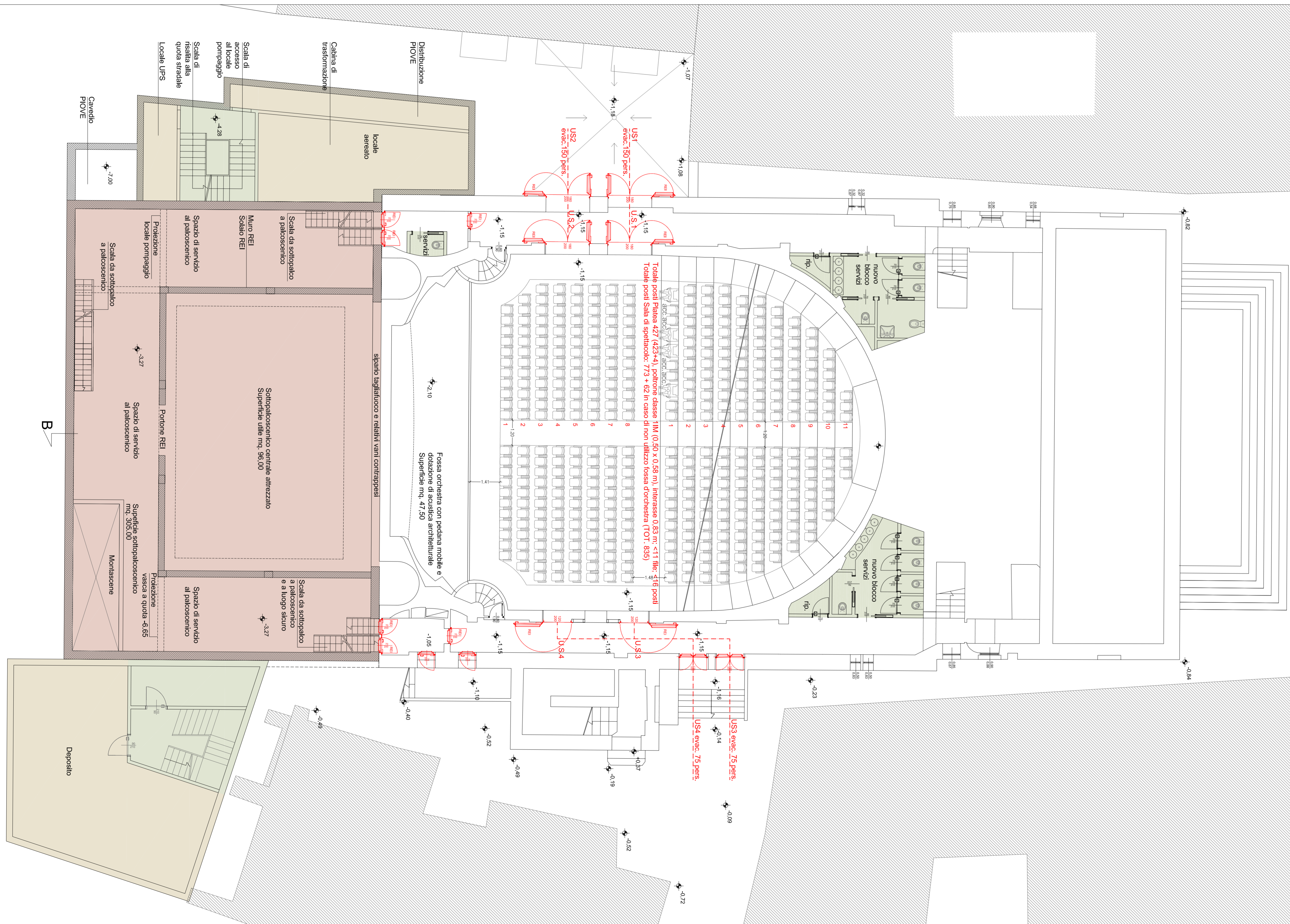
PIANTA A QUOTA SOTTOPALCOSCENICO - SCALA 1:100
