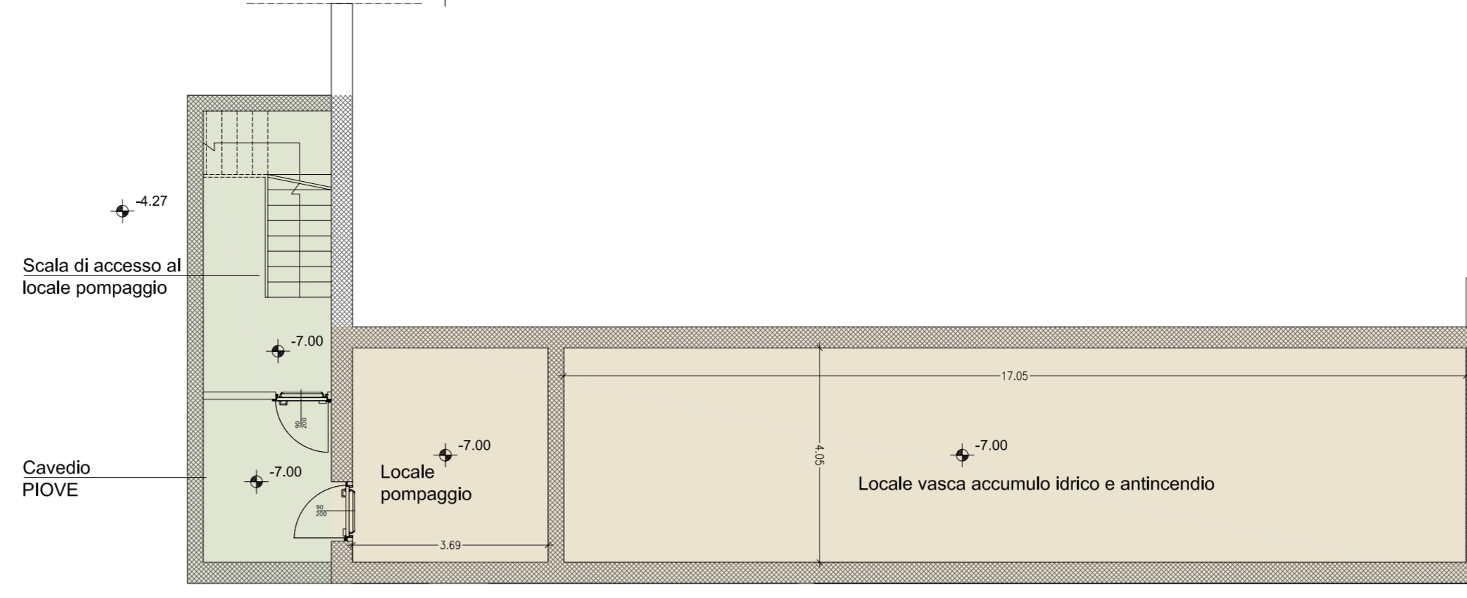
STRALCIO DI PIANTA A QUOTA LOCALE VASCA - SCALA 1:100
